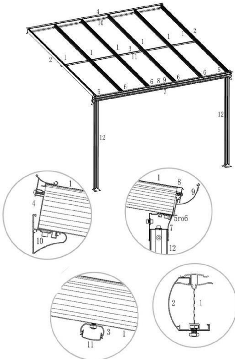
Montageübersicht der Rahmenkonstruktion
